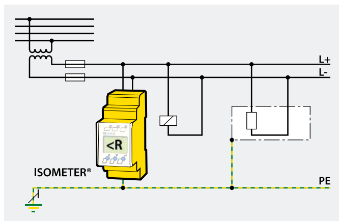
Control de circuito AC con IR420
