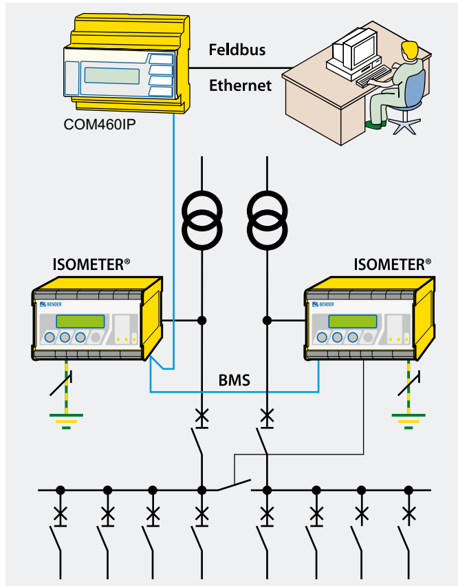
Sistemas IT acoplados
