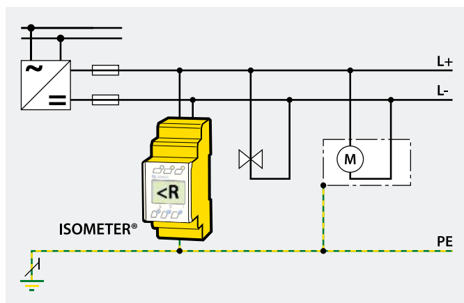
Control de circuito DC con IR425
