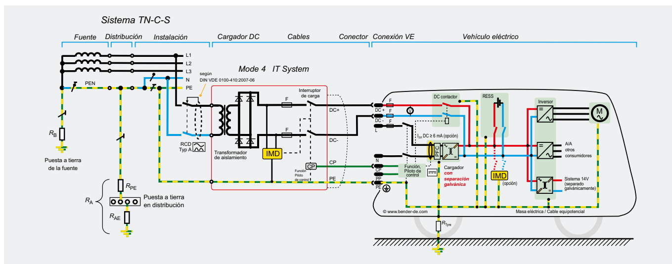
Vigilancia de sistema DC para carga de vehículos con isoEV425
