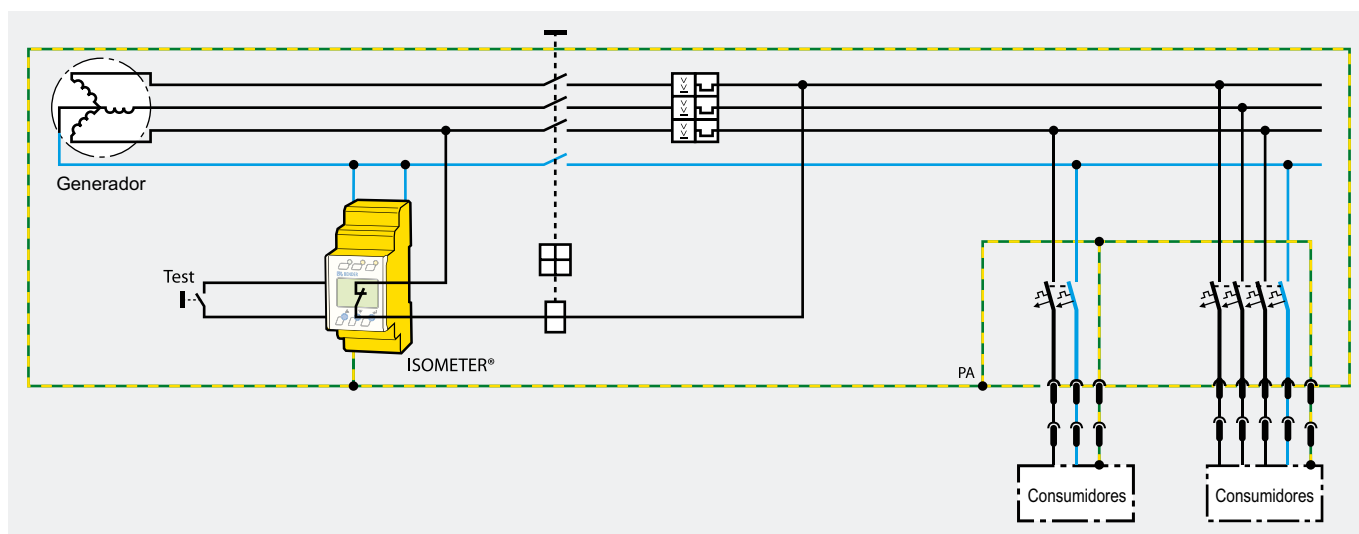
Vigilancia de aislamiento en generadores móviles con IR423
