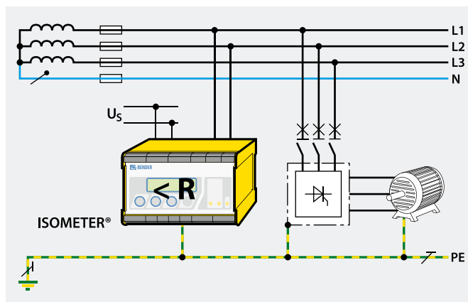
Circuito principal AC/DC con un variador
