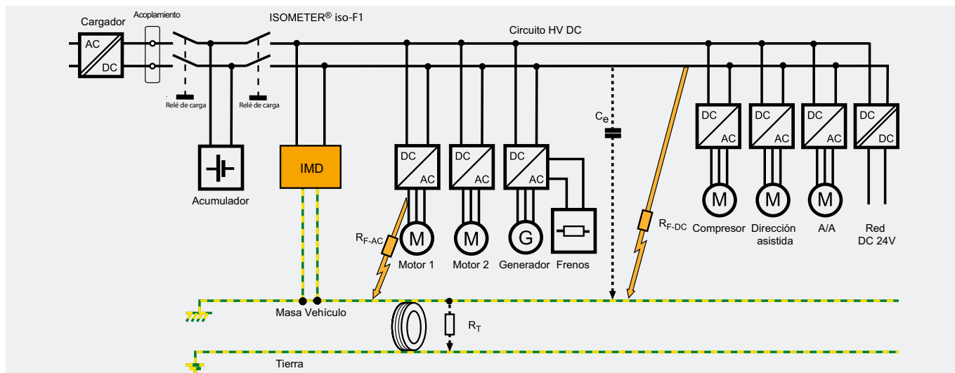
Vigilancia de aislamiento en sistema DC aislado en vehículo con IR155
