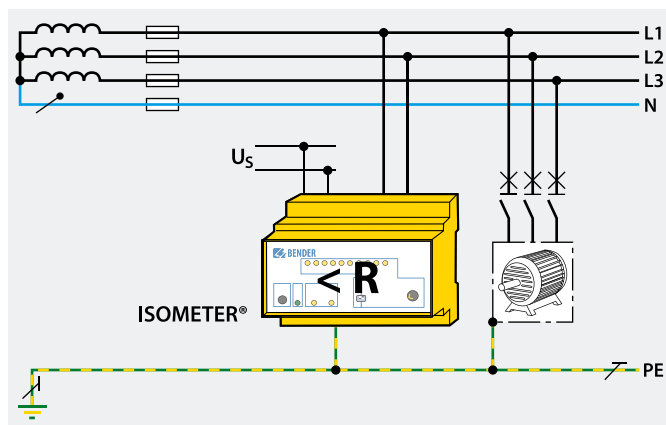
Circuito principal AC con un motor
