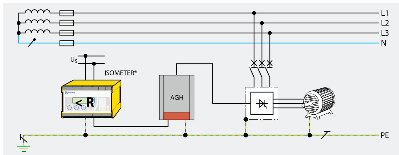
Monitorización de motores de media tensión con IRDH275... y acoplador AGH675S-7
