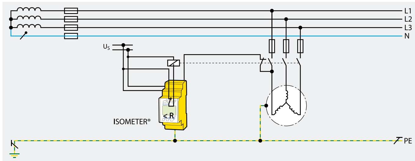
Vigilancia de aislamiento en sistema Offline con IR420-D6 (offline)
