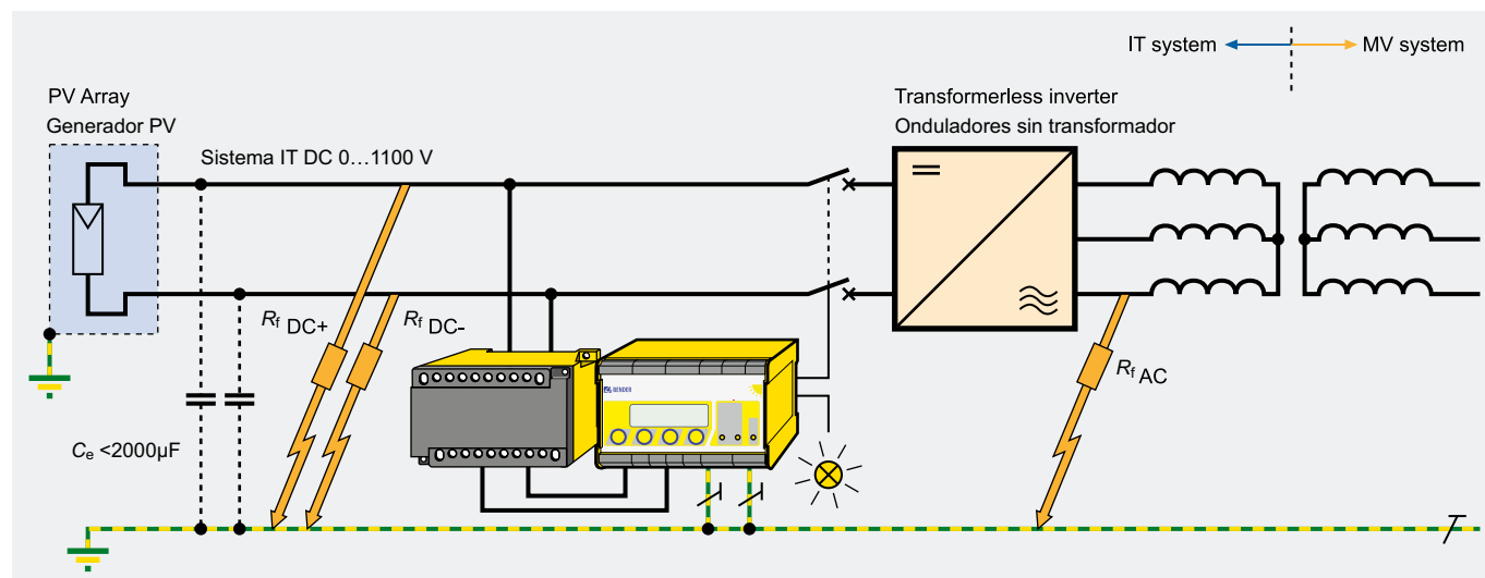
Generadores fotovoltaicos en sistema IT \leq DC 1100 V e ISOMETER® isoPV con acoplador AGH-PV
