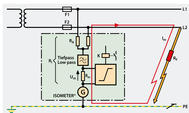
Principio de trabajo ISOMETER®
