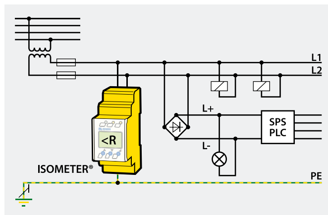
Control de circuito AC/DC con IR425
