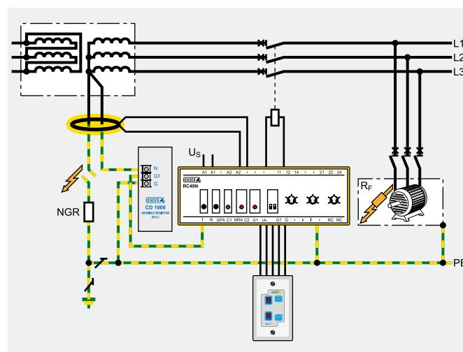
Imagen 3: Vigilancia de fallos a tierra y resistencia de puesta a tierra con RC48N
